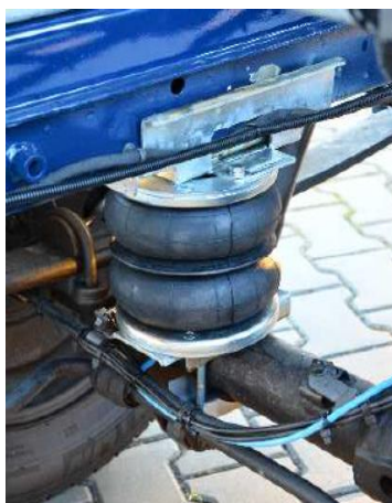
Vzduchové odpružení zadní nápravy
