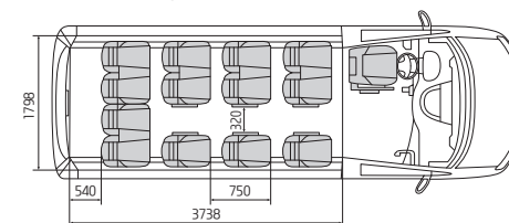
Uspořádání s předními dveřmi
